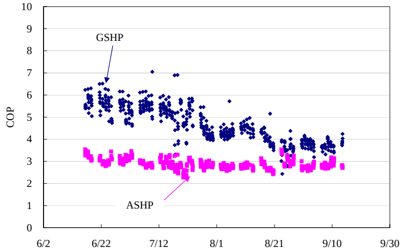
Fig. 10. Units COP
